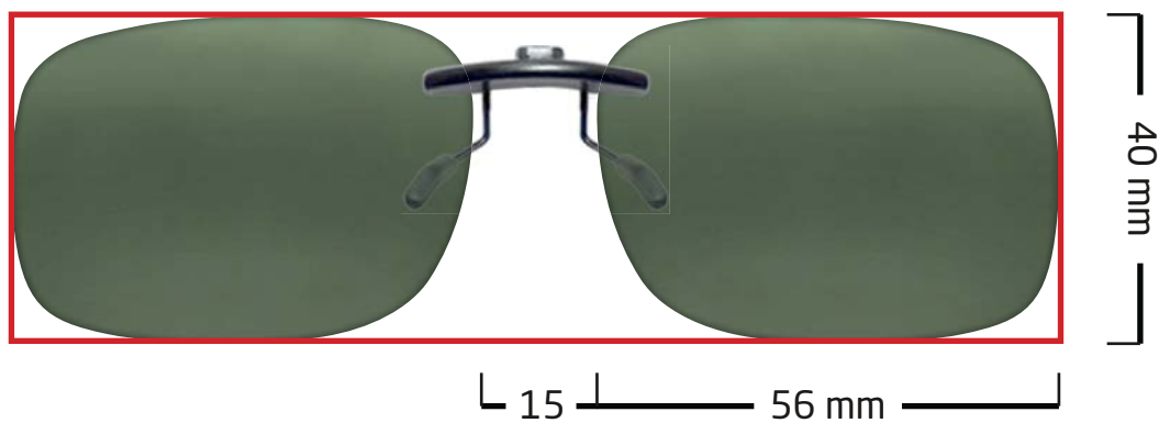
Magiclip SC 670
