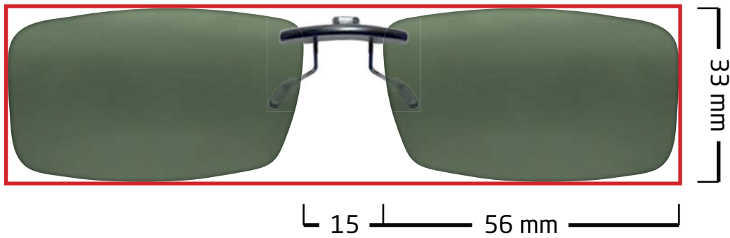
Magiclip SC 304
