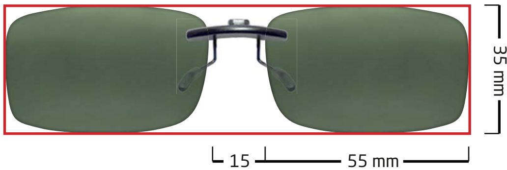
Magiclip SC 313
