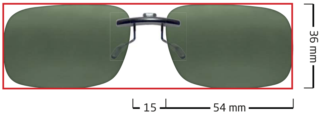
Magiclip SC 669
