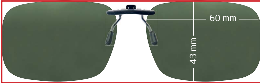
Magiclip SC 301
