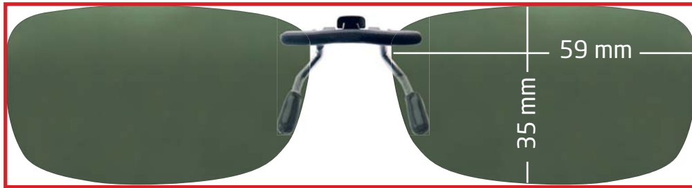
Magiclip SC 306
